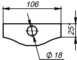
Поз.4 (Ушко) развертка
