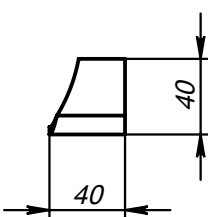
Поз.4 (Ушко)
