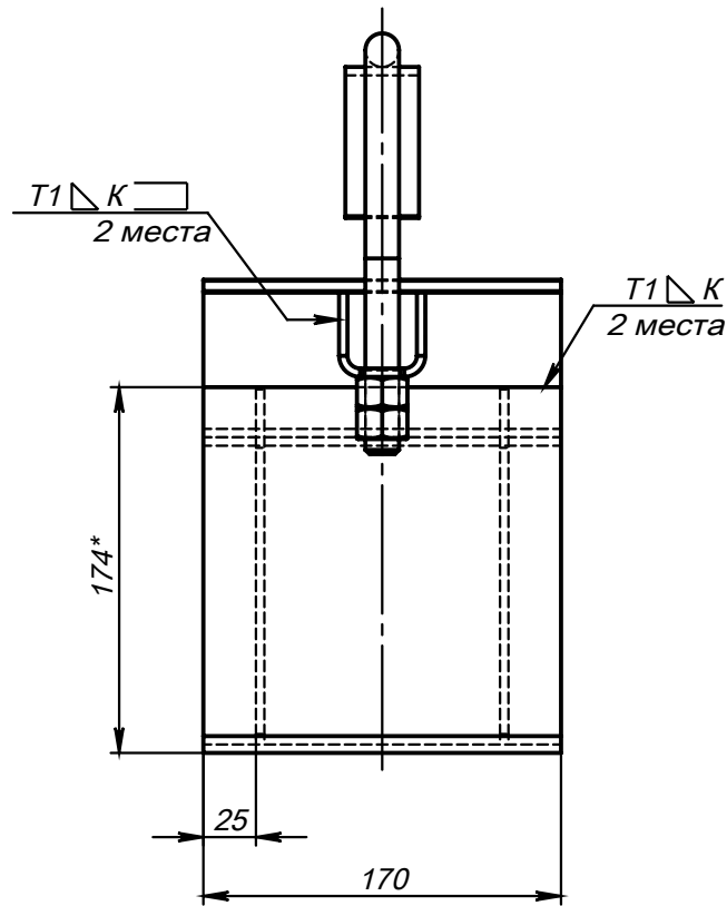
Поз.3 (Ложкемент)
