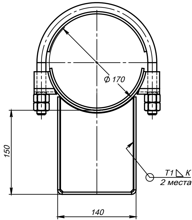
Поз.3 (Ложкемент)
