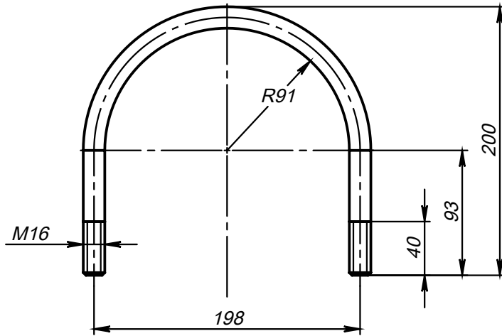
Поз.5 (Хомут)
